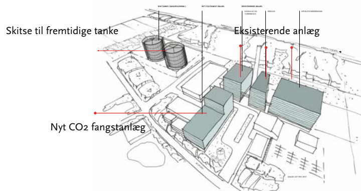
Foreløbig oversigtstegning af det tekniske anlæg i Lisbjerg.
