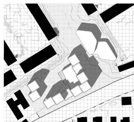
Skyggediagram 21.9. kl. 15 00 1 : 1500
